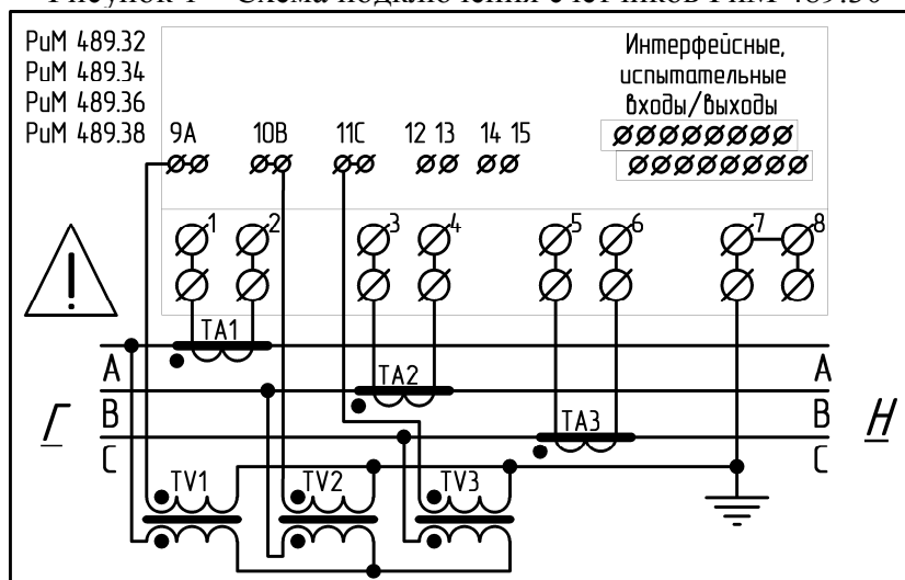
Рисунок 1 – Схема подключения счетчиков РИМ 489.30
