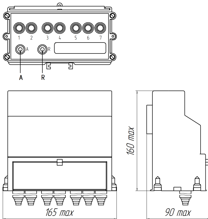
Рисунок 1 – Габаритные, установочные размеры и расположение индикаторов счетчиков
