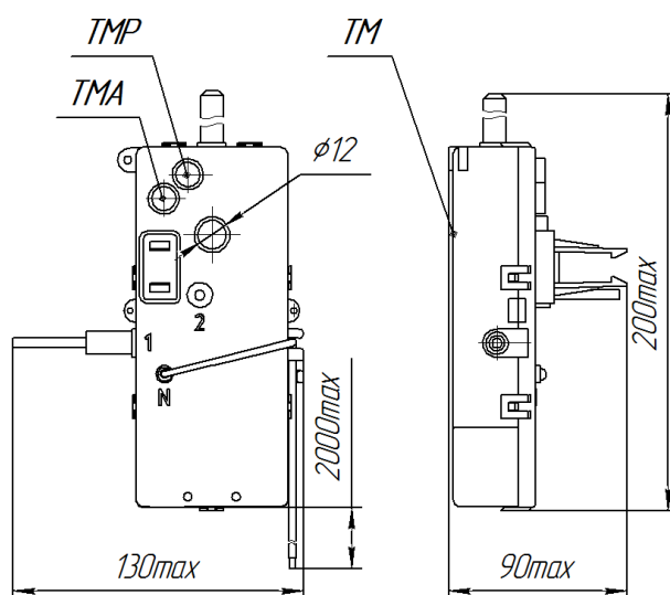
Рисунок 1 – Габаритные, установочные размеры и расположение индикаторов счетчиков (в корпусе тип I)
