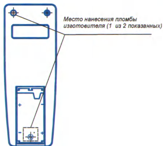
Рисунок 3 – Фотография общего вида и место установки пломбы изготовителя дисплея дистанционного РИМ 040.03
